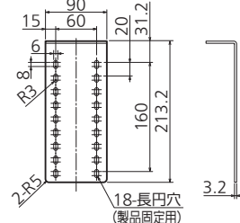
上部振れ止め金具 (別売部品)
