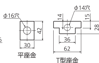
脚固定金具(別売部品)
