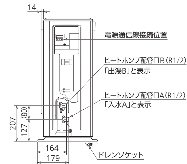
側面図
