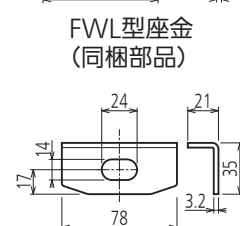
BWL型座金 (同梱部品)
