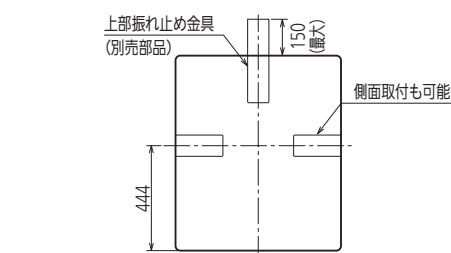
上面図
