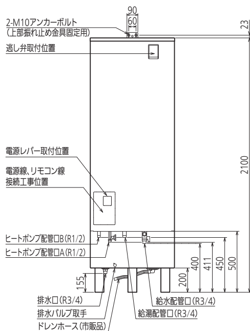
正面図
