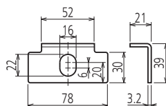
機体脚詳細図
