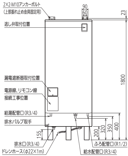
正面図
