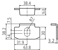
L型座金 (同梱部品)
