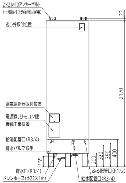
正面図
