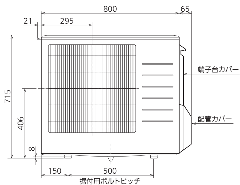
正面図
