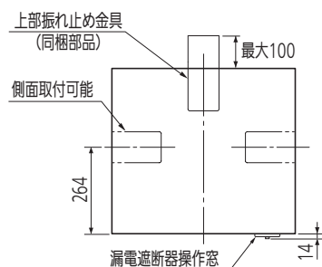
上面図
