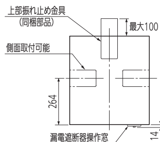
上面図
