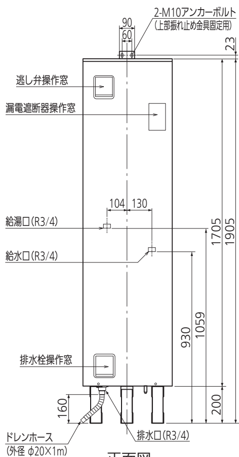
正面図
