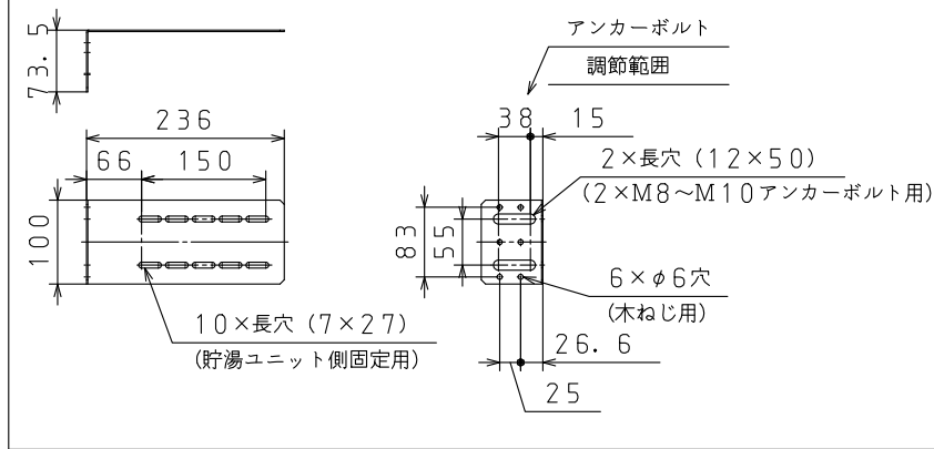
壁固定金具 外形寸法図
