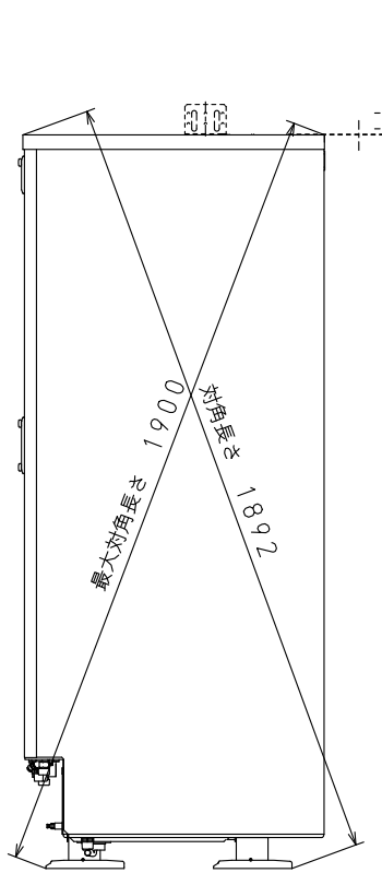
右側面
