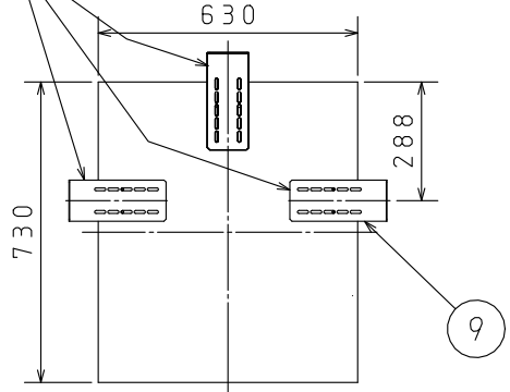
上面
