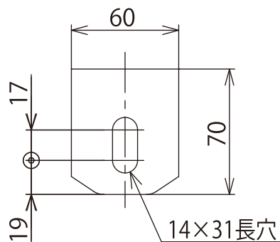
本体中央部脚詳細図
