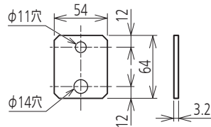
脚固定金具 (同梱部品)
